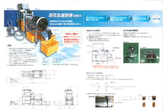
【一般部門】 「落花生選別機（回転式）」
